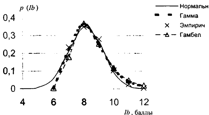
Рис. 6. Примеры использования различных законов распределения вероятностей для аппроксимации повторяемости торнадо разной разрушительной силы
