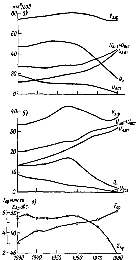
Рис. 7. Динамика значений водных ресурсов в зоне формирования U_{3.ф} стока в замыкающем створе Q_H , естественных U_{ест} и антропогенных U_{ант} потерь стока для р. Амударья — Чатлы (а) и р. Сырдарья — Казалинск (б), уровней Аральского моря и суммарных площадей в его бассейне (в)
