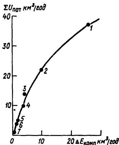
Рис. 6. Зависимость объема „компенсационных ресурсов“ \Delta E_{\text{комп}} от суммарных потерь стока в бассейне \Sigma U_{\text{пот}} . Цифры — номера бассейнов по табл. 8.
