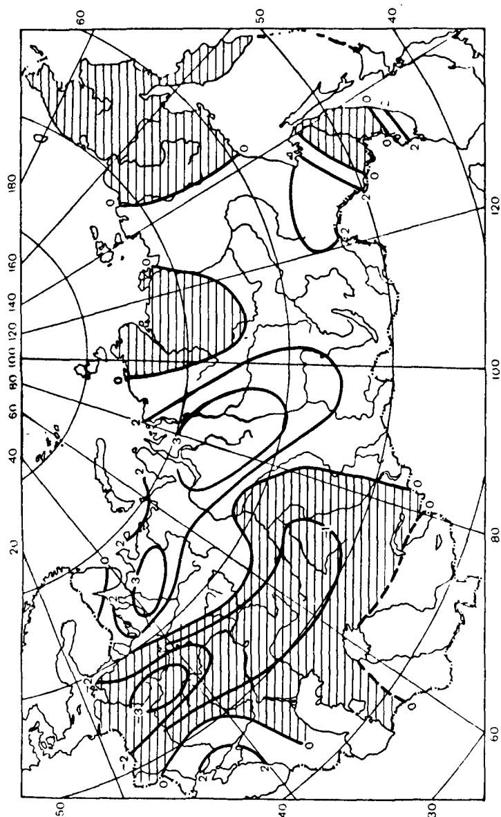
Рис. 31. Изменение среднего годового стока рек СССР (в см слон) при повышении глобальной температуры воздуха на 0,5 °С. (на 1990 г.).
