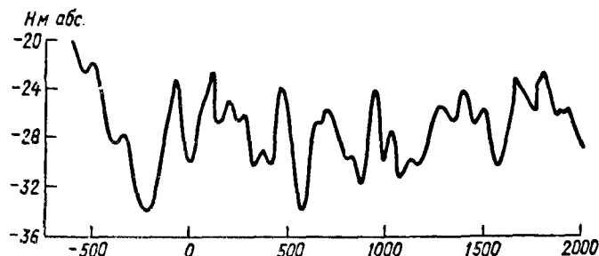
Рис. 13. Изменение уровня Каспийского моря за последние 2,0–2,5 тыс. лет (по Р. К. Клиге).
