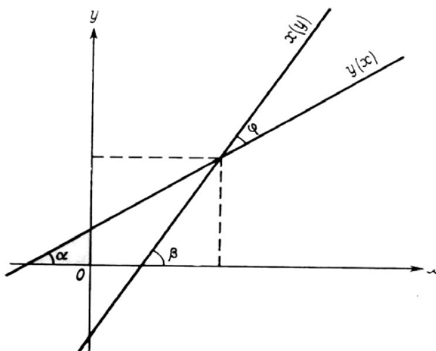
Рисунок П.10 – Прямые регрессии x(y) и y(x) .
