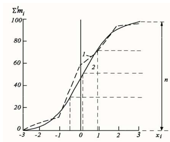
Рисунок П.3 – Огива (1) и интегральная кривая распределения (2).
