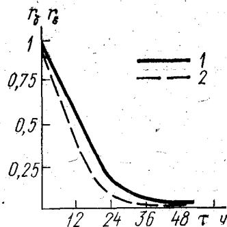
Рис. 7.3. Коэффициенты автокорреляции временных рядов оценок \delta(1) и \epsilon(2) . По оси абсцисс отложен сдвиг по времени \tau в часах
