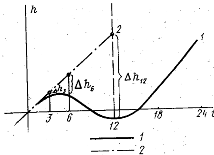
Рис. 5.4. Влияние выбора шага по времени на результат экстраполяции хода величины h :
