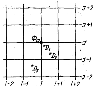
Рис. 8.1. Расположение трех пунктов, в которых предполагается создать метод локального прогноза величины D на основе модельной статистики по данным поля \Phi_{xj} , представленного на регулярной сетке, где I, j — соответственно номера столбцов и строк
