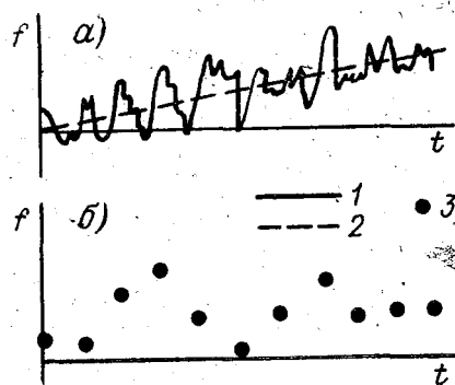
Рис. 3.1. Образование фиктивных крупномасштабных колебаний под влиянием дискретности системы наблюдений. Смесь сигнала и шума (1), налагающегося на истинный сигнал (2) приведены в части (а), наблюдаемые значения (3) — в части (б)
