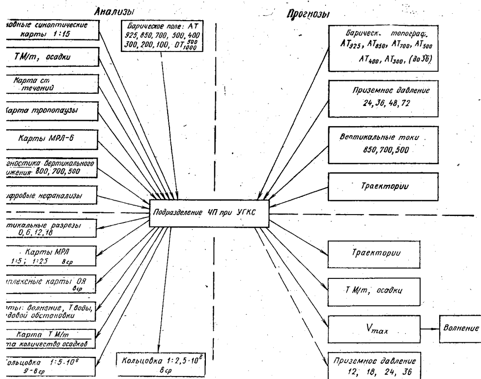
Рис. 2.1. Аэросинооптические материалы, поступающие в территориальные ГМЦ и вырабатываемые в подразделениях численного прогноза (ЧП).
