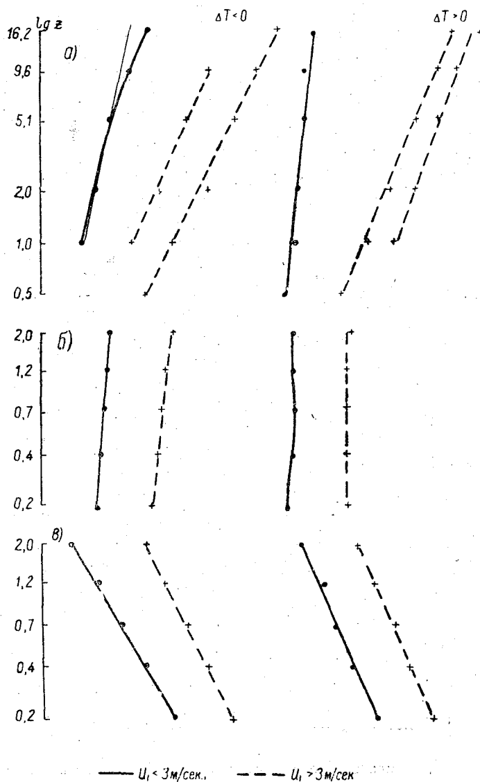
Рис. 1. Распределение метеозлементов над Цимлянским водохранилищем.
