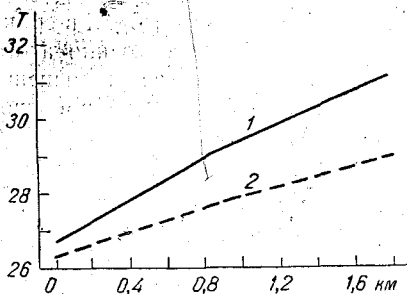
Рис. 3. Изменение температуры по горизонтали при неустойчивой стратификации (8 серий).
