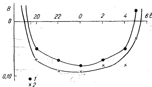
Рис. 4. Изменение радиационного баланса в течение ночи. 1 — вода, 2 — суша.
