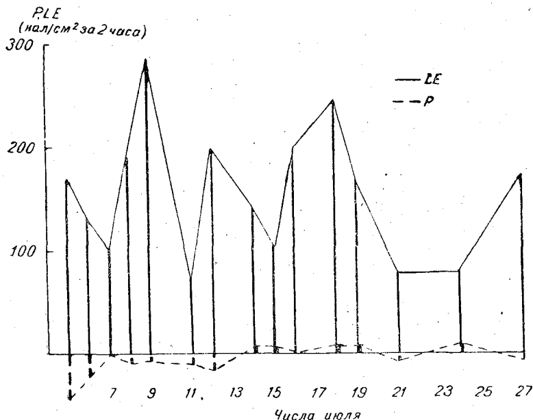
Рис. 1. Ход величин турбулентного потока тепла и затрат тепла на испарение в июле 1954 г.
