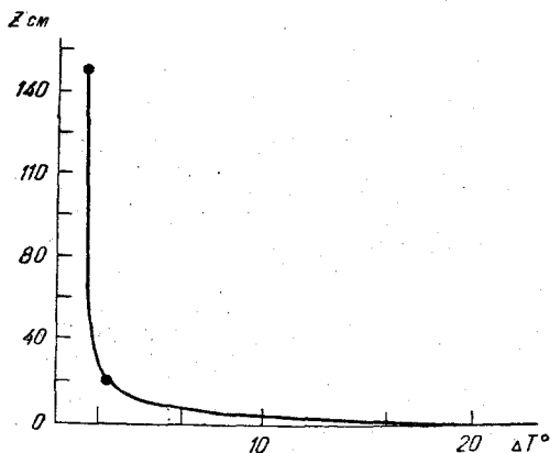
Рис. 6. Зависимость горизонтальной разности температур от высоты.
