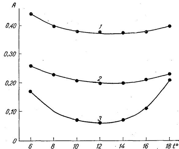
Рис. 1. Дневной ход альбедо. 1 — песок, 2 — трава, 3 — вода.
