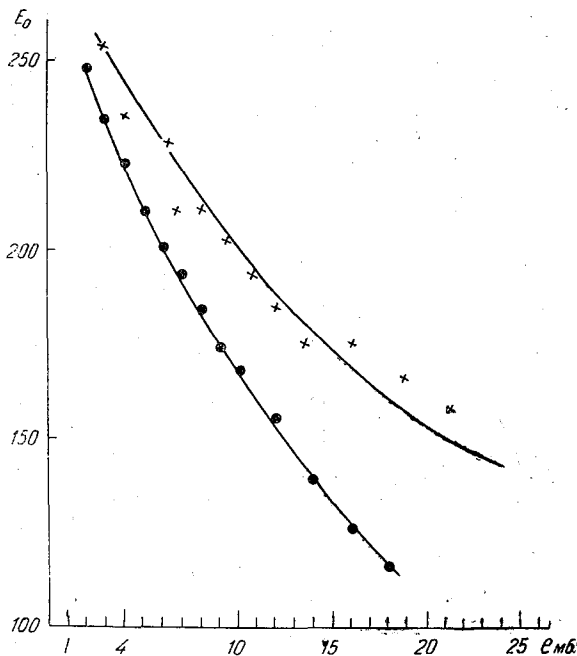
Рис. 3. Зависимость эффективного излучения от влажности.
