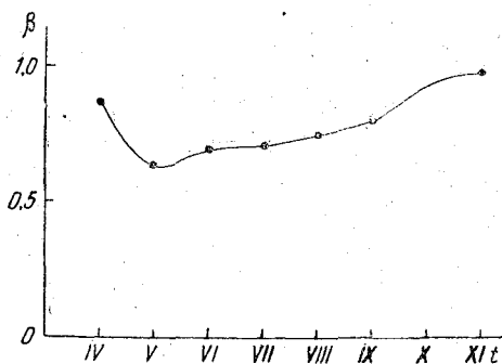
Рис. 1. Временной ход коэффициента \beta (средний для водоемов).
