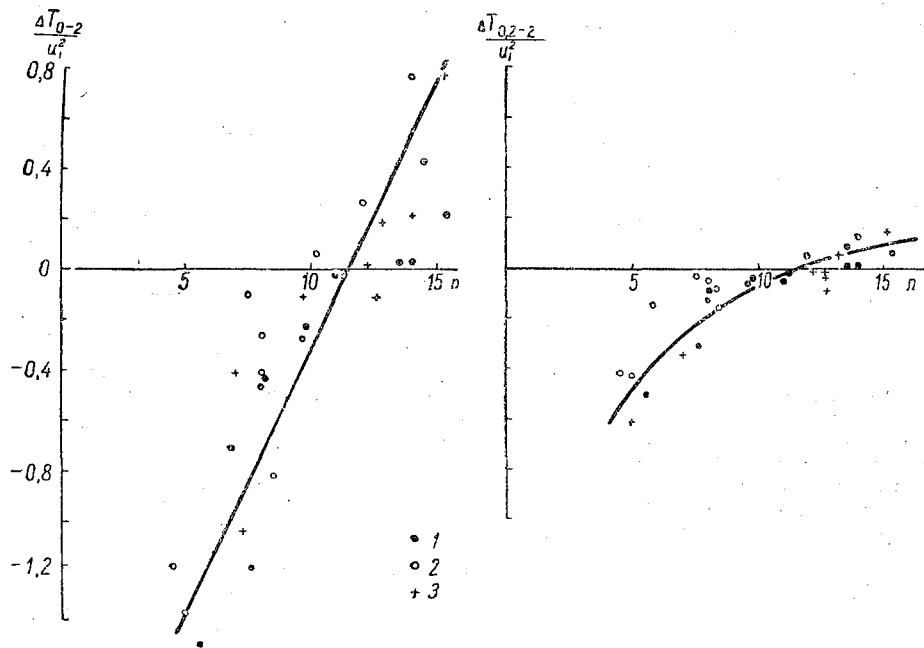
Рис. 3. Связь n с \frac{\Delta T_{0,2} - 2}{u_1^2} и с \frac{\Delta T_{0,2-2}}{u_1^2} .
