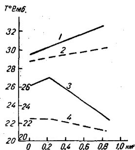
Рис. 2. Измерение температуры и влажности воздуха у берега 2/VII в 12 ч. 1 — температура 20 см, 2 — температура 150 см, 3 — влажность 20 см, 4 — влажность 150 см.
