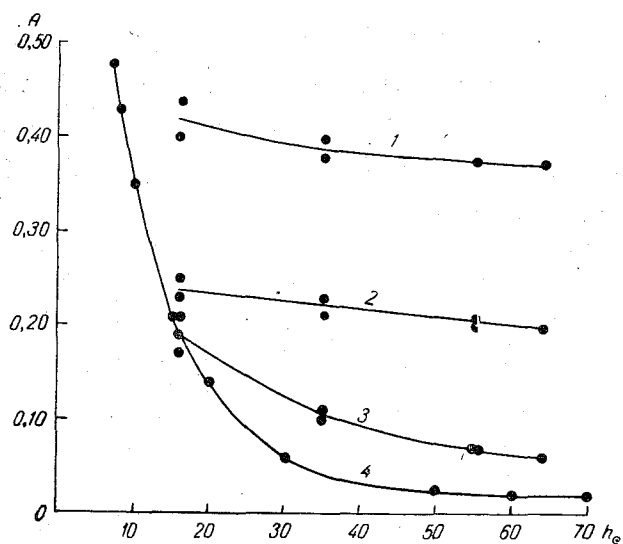
Рис. 2. Зависимость альbedo от высоты солнца.
