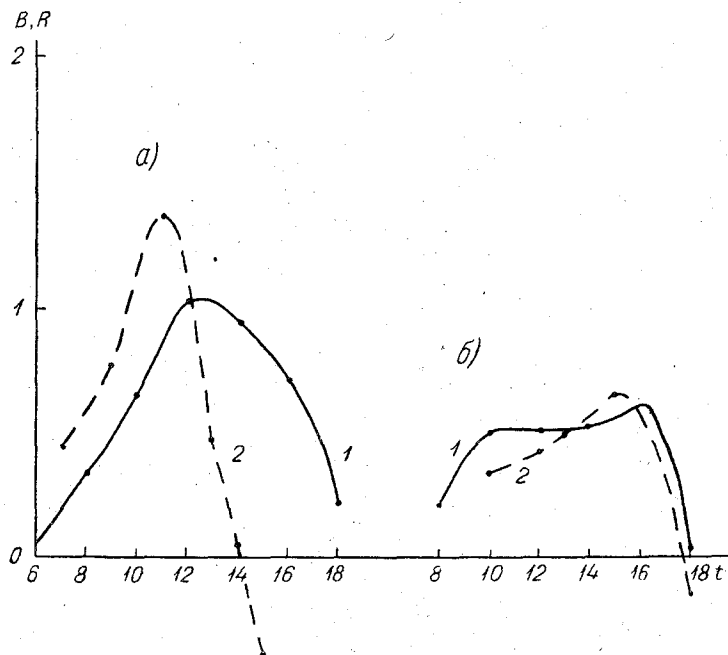
Рис. 6. Теплообмен в воде и радиационный баланс за 21/VII (а) и 23/VII (б) 1954 г.
