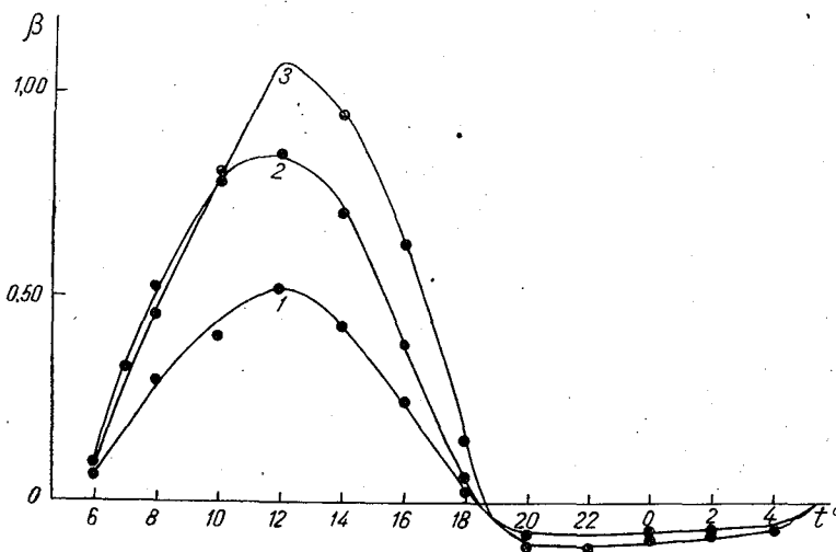
Рис. 3. Суточный ход радиационного баланса. 1 — песок, 2 — трава, 3 — вода.
