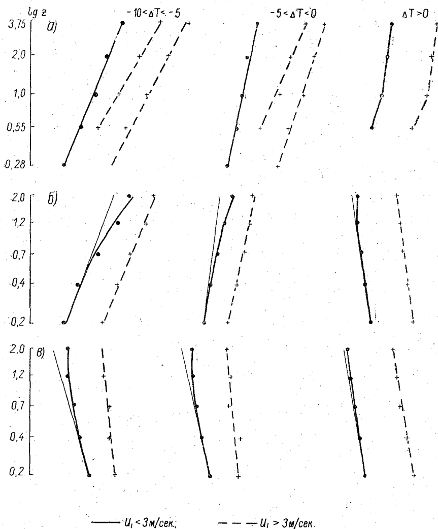
Рис. 2. Распределение метеоэлементов над оз. Красавица.
