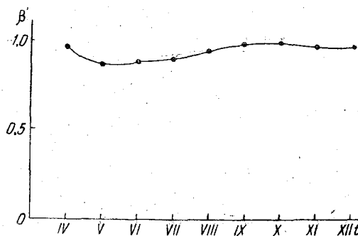
Рис. 2. Временной ход коэффициента \beta (средний для водоемов).
