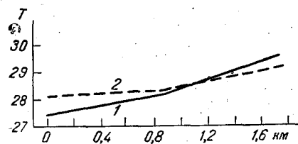
Рис. 5. Изменение температуры воздуха по горизонтали при устойчивой стратификации. 1 — 20 см, 2 — 150 см.
