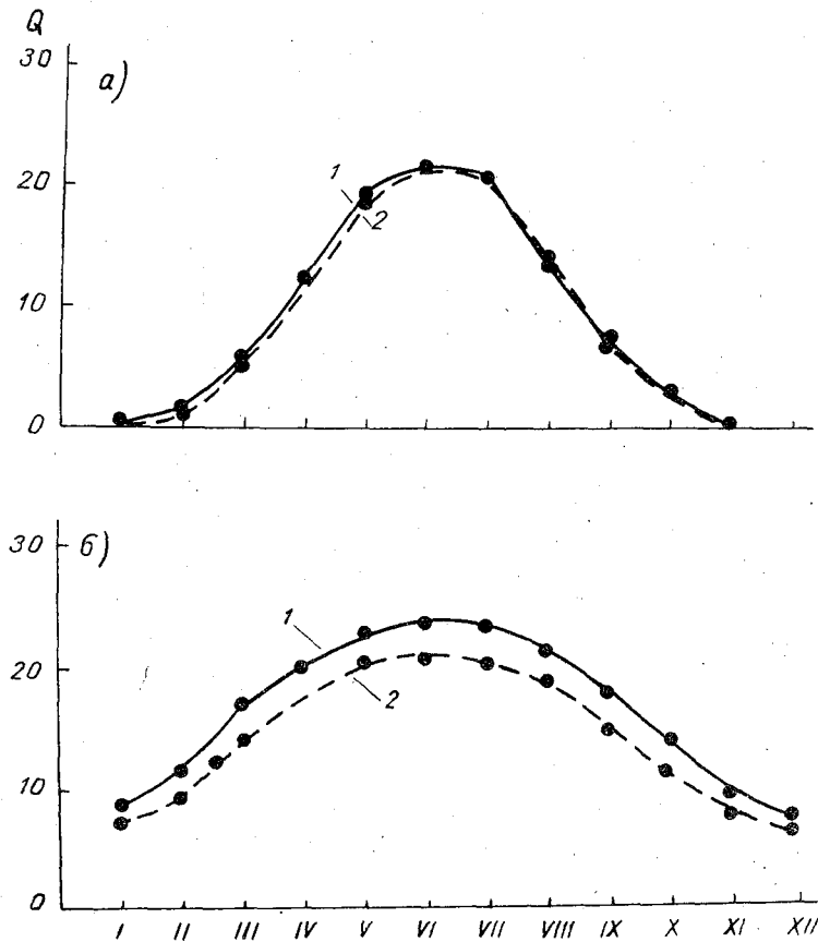
Рис. 1. Годовой ход суммарной радиации при безоблачном небе: a — широта 70^\circ , b — широта 40^\circ . 1 — по ф-ле Берлянд, 2 — по ф-ле Браславского.
