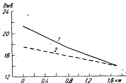
Рис. 7. Изменение влажности воздуха по горизонтали при неустойчивой стратификации.
