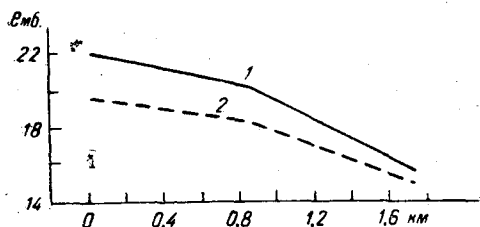
Рис. 8. Изменение влажности по горизонтали при устойчивой температурной стратификации атмосферы.
