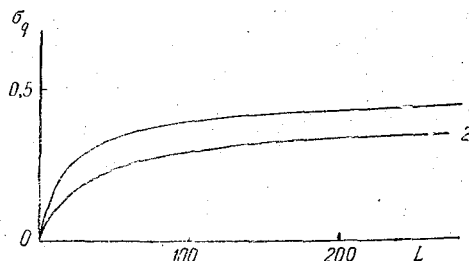
Рис. 1. Зависимость величины \sigma_q от размера водоема.
