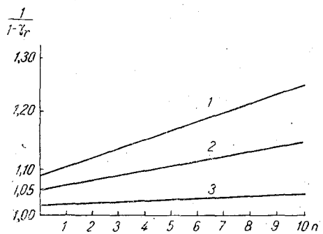
Рис. 2. Зависимость величины k_r от степени облачности. 1 — при r = 0.25 , 2 — при r = 0.15 , 3 — при r = 0.05 .
