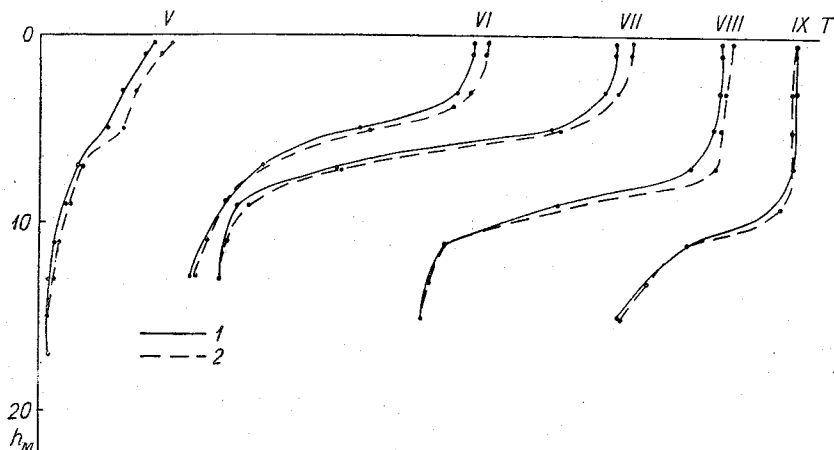
Рис. 1. Профили температуры воды по среднемесячным данным.
