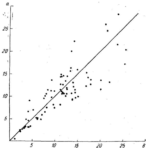
Рис. 2. Связь правой и левой частей выражения (8) для влажности.
