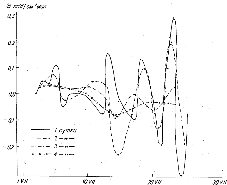
Рис. 7. Величины тепловых потоков в воду на Цимлянском водохранилище, рассчитанные за различные интервалы времени.
