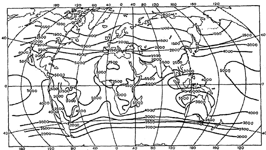
Рис. 53. Радиационный баланс земной поверхности за год (МДж/м²).
