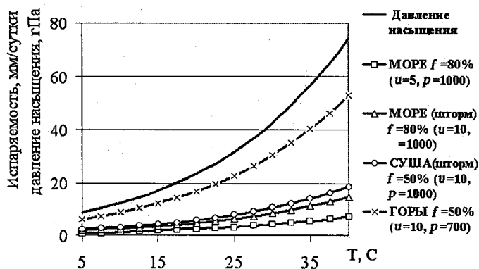
Рис.22. Испаряемость в различных условиях.
