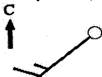
Рис. 76. Обозначение юго-западного ветра, дующего со скоростью 7,5 м/с.
