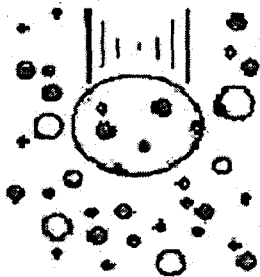
Рис. 27. Рост капель за счет коагуляции.
