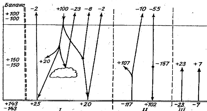
Рис.106. Тепловой баланс земной поверхности и атмосферы.
