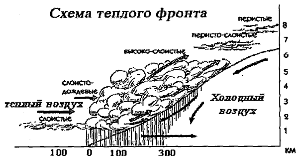
Рис.97. Движение воздуха, облачность и осадки при прохождении фронтов.
