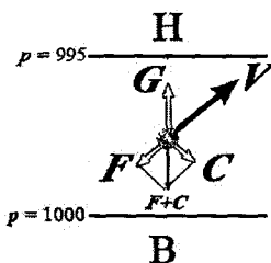
Рис. 82. Расположение относительно вектора скорости V движения частицы сил, действующих на нее в слое трения. Обозначения: G – сила барического градиента, C – сила Кориолиса, F – сила трения. F+C – равнодействующая сил трения и Кориолиса, B – область повышенного давления, H – область пониженного давления.
