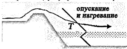
Рис. 74. Формирование инверсий оседания.
