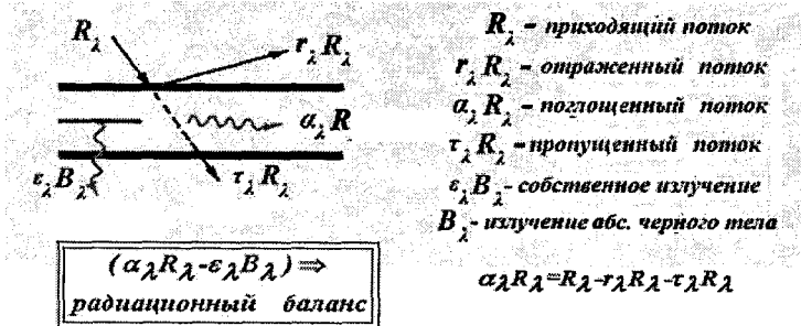
Рис.35. К определению понятия радиационный баланс.
