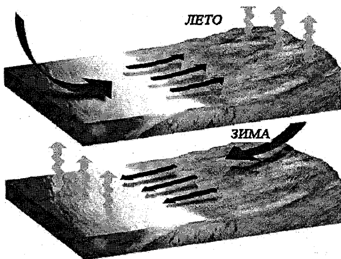
Рис. 94. Схема смены направления приземных ветров при муссонной циркуляции над Индией.
