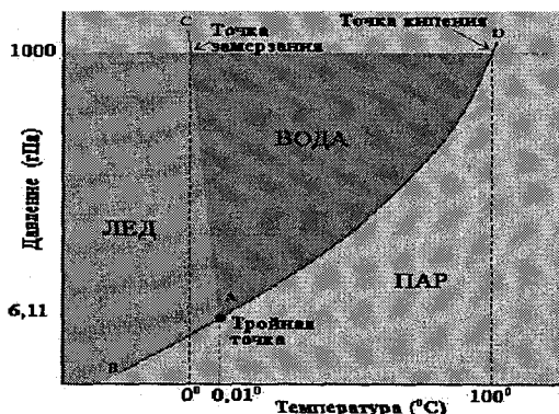
Рис. 21. Диаграмма фазового состояния воды.
