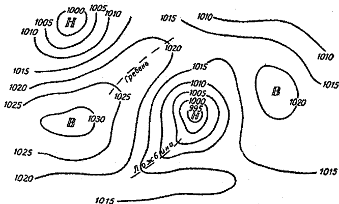
Рис. 10. Изобары поля давления. Н — циклоны, В — антициклоны.
