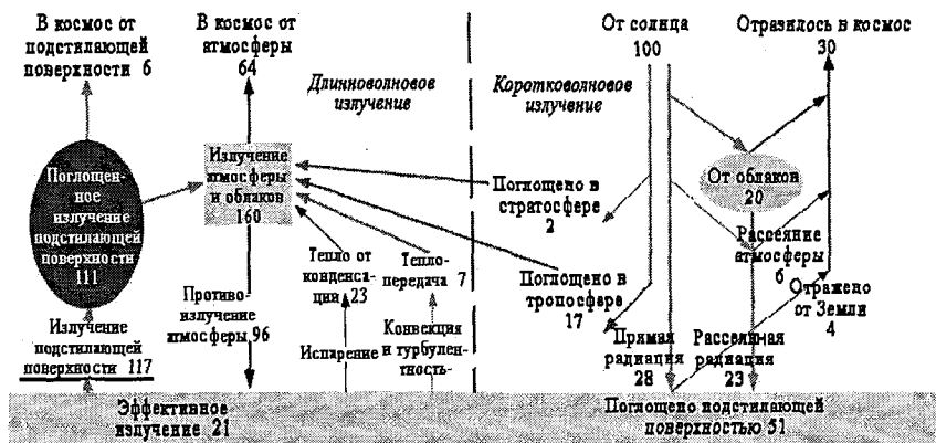
Рис. 54. Радиационный и тепловой балансы системы Земля – атмосфера и отдельных ее частей.
