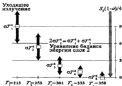
Рис. 50. Поток радиации в атмосфере, состоящей из трех полностью поглощающих длинноволновое излучение слоев.
