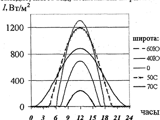
Рис.39. Суточный ход инсоляции на разных широтах.
