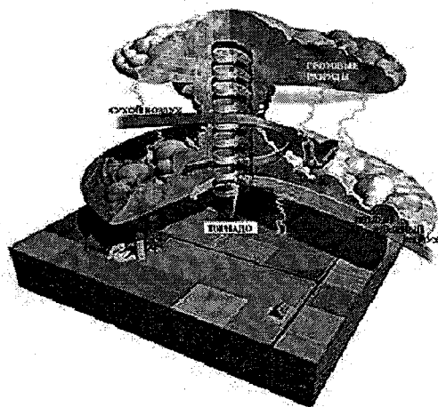
Рис. 91. Схема кучево-дождевого облака, в котором возникло торнадо.
