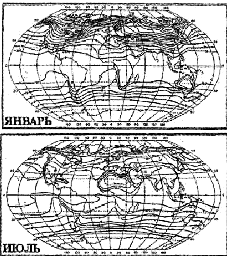
Рис. 13. Среднее распределение температуры воздуха на уровне моря.
