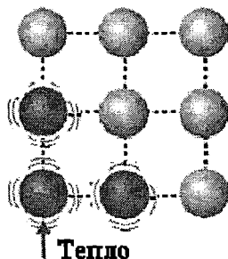
Рис. 57. Механизм теплопроводности в твердых телах (колебания атомов кристаллической решетки).
