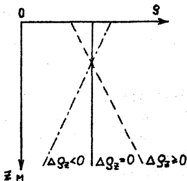
Рис. 3.1. Типы изменения плотности воды с глубиной.
