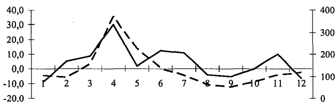
Рис. 7.13. Статистические характеристики ряда уровней малого озера Сенно с умеренным водообменом до фильтрации (а) и после (б)
