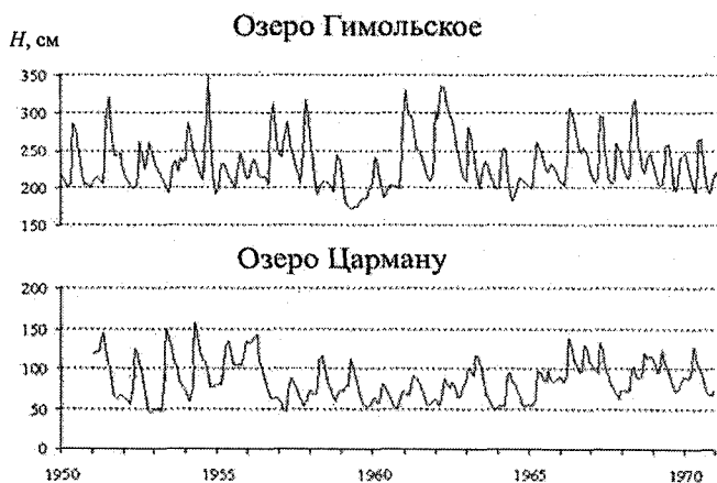
Рис. 7.10. Средние месячные уровни большого и среднего озера с умеренно-сильным водообменом
