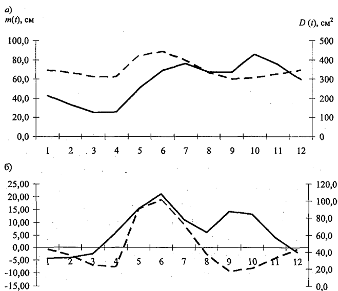
Рис. 7.14. Статистические характеристики ряда уровней большого озера Сязозеро с умеренным водообменом до фильтрации (а) и после (б)
