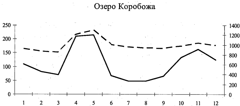
Рис. 7.12. Статистические характеристики рядов уровней больших озер с сильным водообменном
