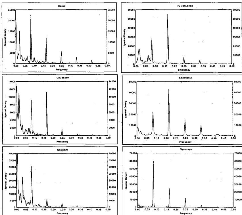
Рис. 7.16. Оценка спектральной плотности уровней колебаний озер разных классов водообмена
