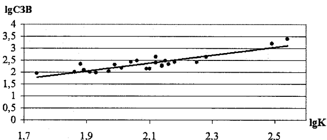
Рис. 3.1. Зависимость количества сброшенных загрязненных сточных вод в водные объекты крупных городов России (СЗВ) от коэффициента антропогенного давления (K)
