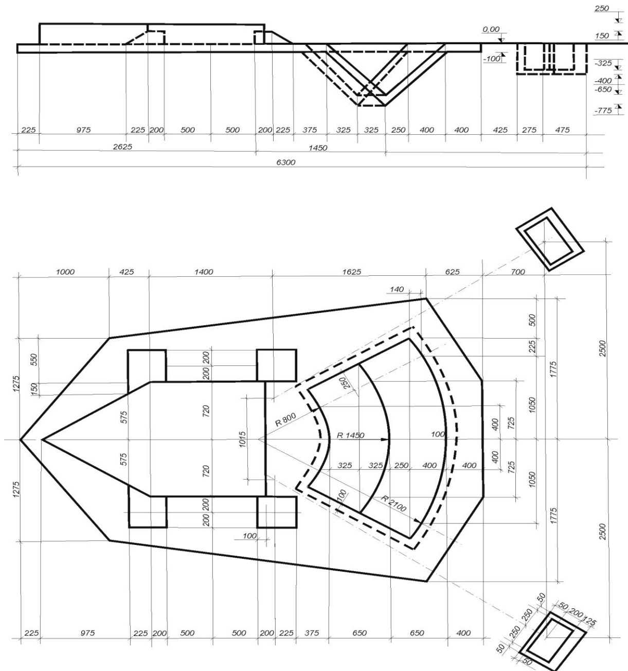
Рисунок 4 – Схема стационарной ОП
