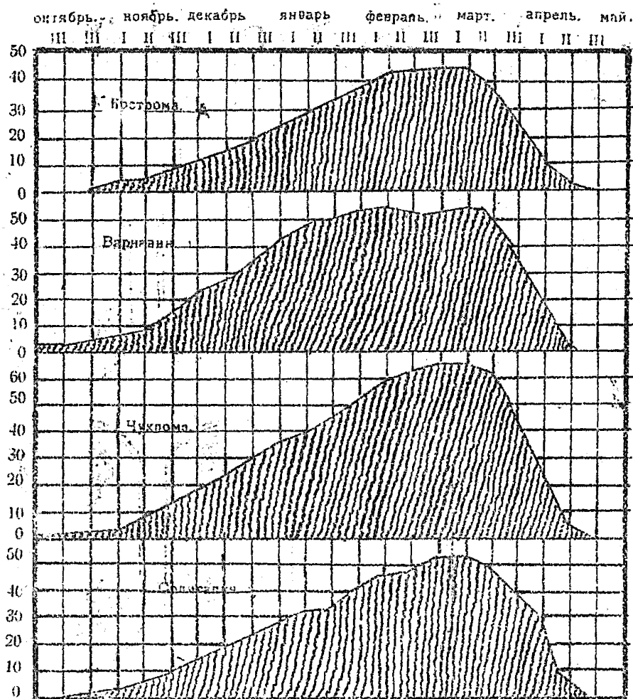
Средняя толщина снегового покрова по декадам.
