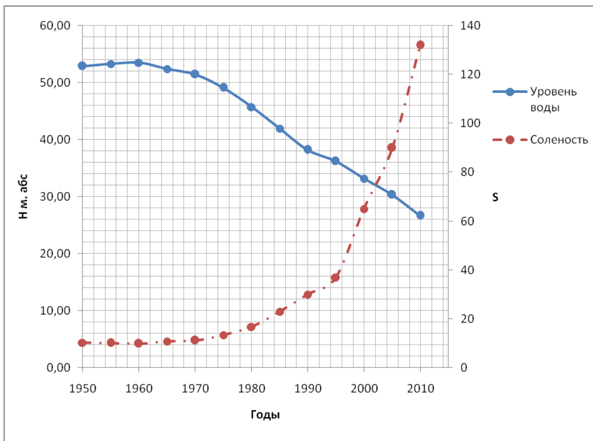
Рис 18. График зависимости уровня и солёности Аральского моря.
