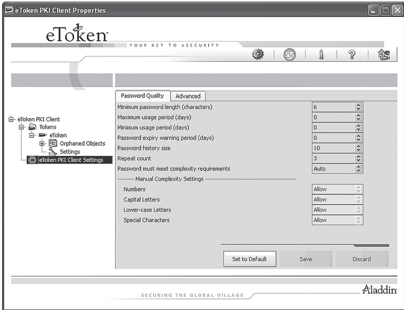
Рис. 5. Окно настройки пароля eToken
