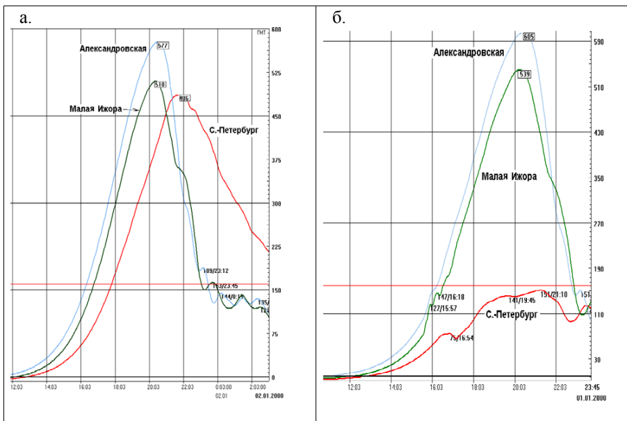
Рис. 6. Временной ход уровня в Александровской, Малой Ижоре и СПб при прохождении экстремального циклона вдоль 61.5 с.ш. со скоростью 50 км/час. КЗС в проектном состоянии. Слева – КЗС открыт, справа: закрыт с момента перехода уровня у КЗС со стороны Финского залива через отметку 1 м
