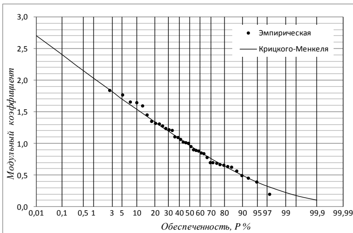
Рис. 7. Эмпирическая и аналитическая кривые обеспеченностей среднегодовых расходов воды в модульных коэффициентах, р. Лжа – д. Фелицианово (расчет по удлинненному ряду; Q_{\text{ср}} = 3,89 , C_v = 0,40 , C_v/C_v = 1 ).
