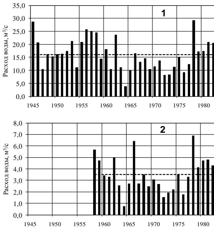
Рис.1 – Хронологические графики среднегодовых расходов воды; 1 – р. Утря – д. Большая Губа (река-аналог); 2 – р. Лжа – д. Фелицианово (расчетная река).
