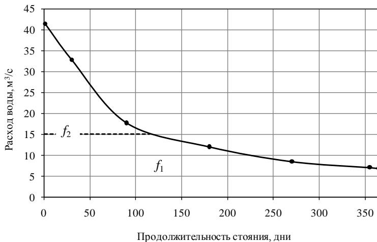
Рис.4. Кривая продолжительности стояния суточных расходов, р. Луга – ст. Толмачево; 1973 – маловодный год; Q_{cp} = 15,0 \text{ м}^3/\text{с} ; \varphi = 0,87 .
