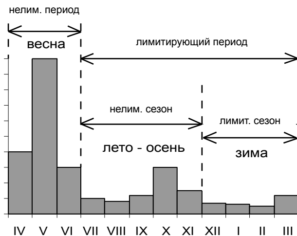
Рис.1. Схема разбивки водохозяйственного года на сезоны и периоды при расчете внутригодичного распределения стока.
