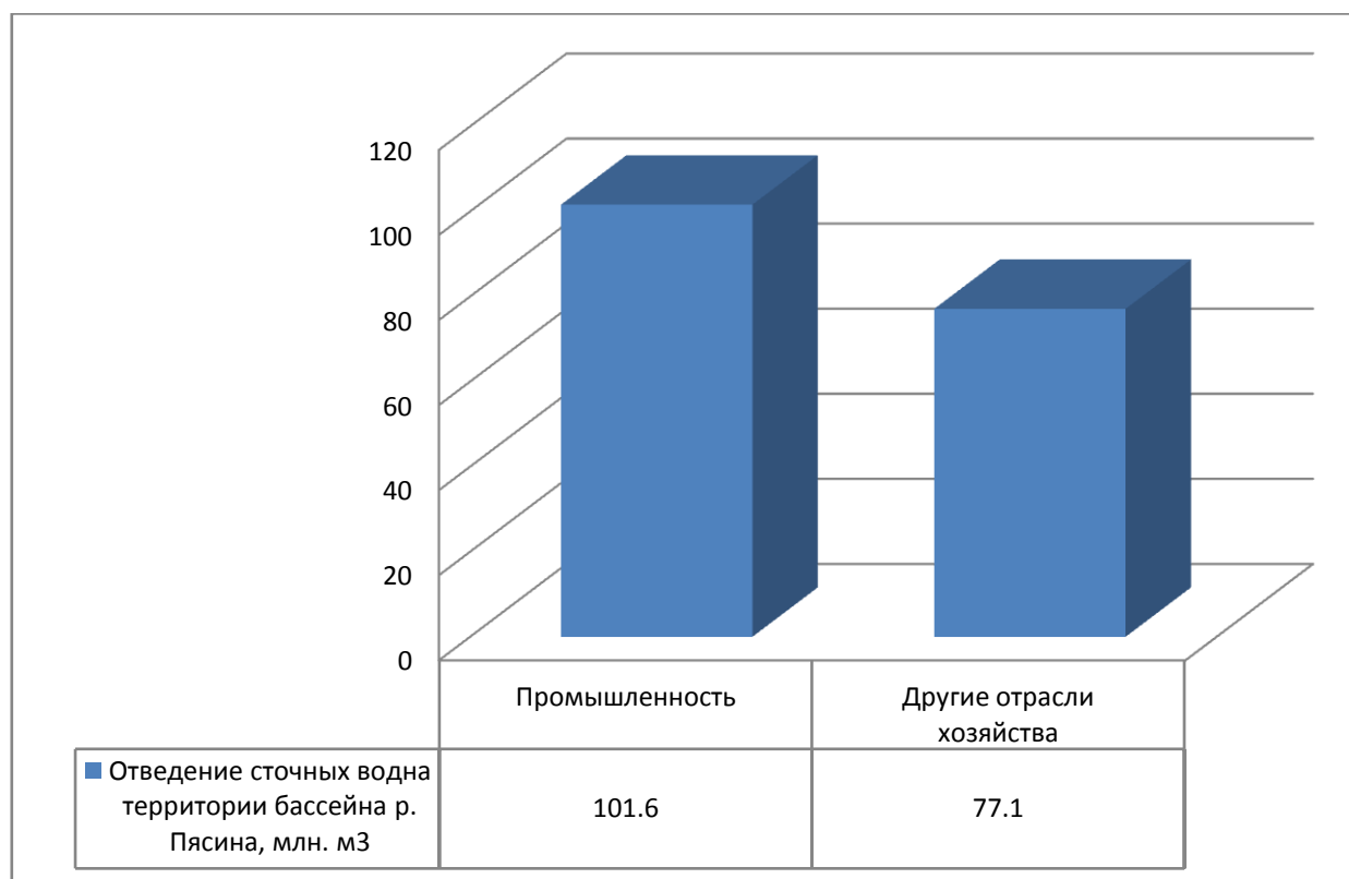
Рисунок 9 – Отведение сточных вод в водные объекты в промышленности, млн. м 3 (усредненные данные за период 2001-2010 гг.)
