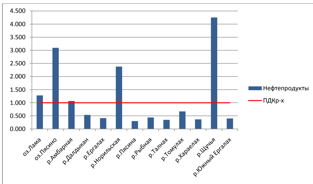
Рисунок 6 – Превышение ПДК рх по содержанию в воде водных объектов нефтепродуктов
