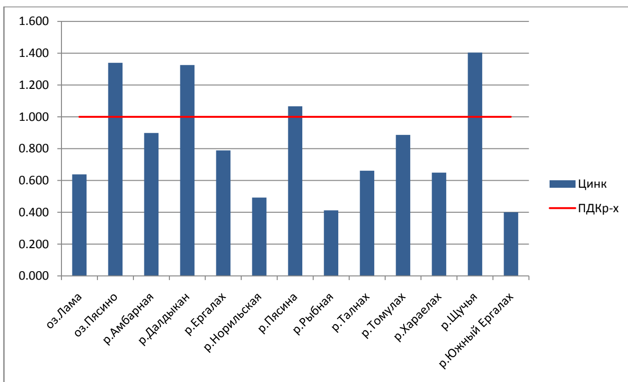
Рисунок 4 – Превышение ПДК рх по содержанию в воде водных объектов цинка
