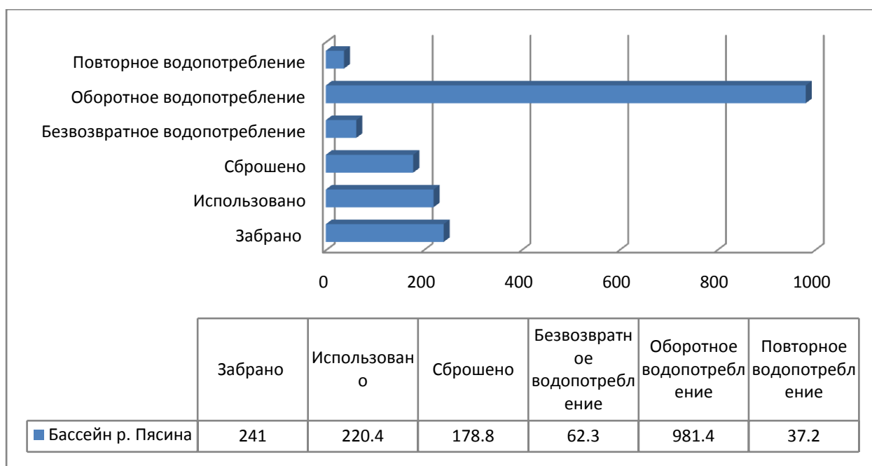
Рисунок 3 – Способы использования водных объектов в бассейне р. Пясины, млн. м 3 (усредненные данные за период 2001-2010 гг.)
