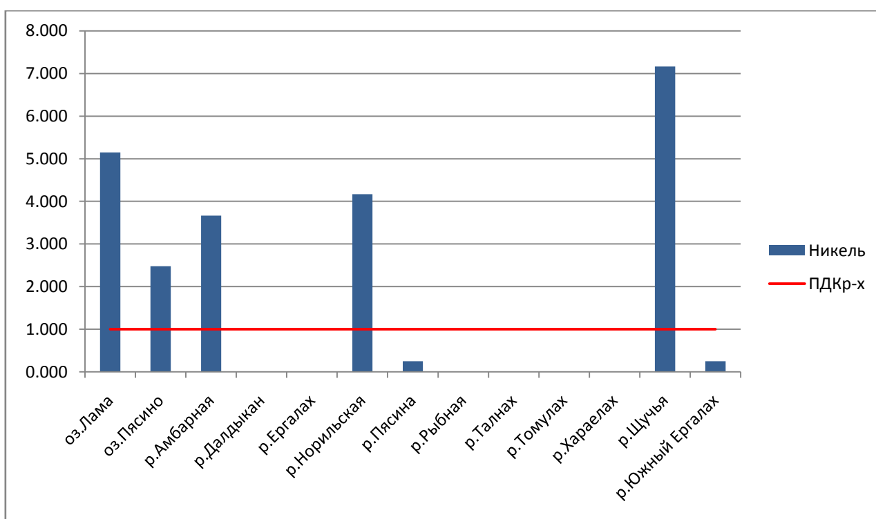
Рисунок 5 – Превышение ПДК рх по содержанию в воде водных объектов никеля
