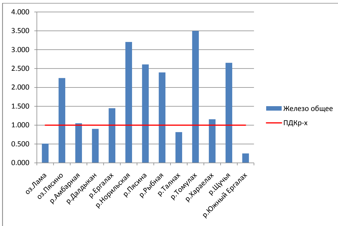
Рисунок 2 – Превышение ПДК рх по содержанию в воде водных объектов железа
